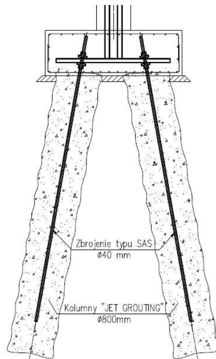
PRZEKRÓJ PRZEZ STOPE FUNDAMENTOWĄ
