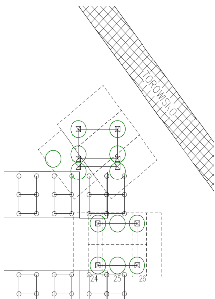
ROZMIESZCZENIE KOLUMN „JET GROUTING” POD TYMCZASOWYMI PODPORAMI
