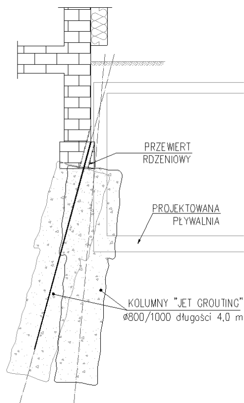
KONSTRUKCJA KOLUMN „JET GROUTING”
